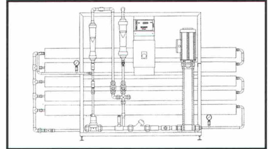
DELTA MC Tipi Ters-Osmoz Cihazı Planı (Delta MC 60-140 modelleri için)
